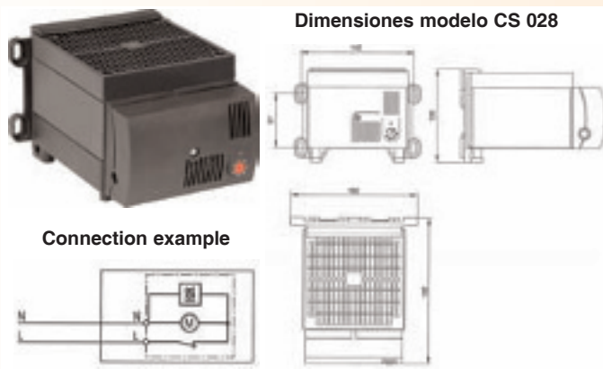
Dimensiones modelo CS 028
